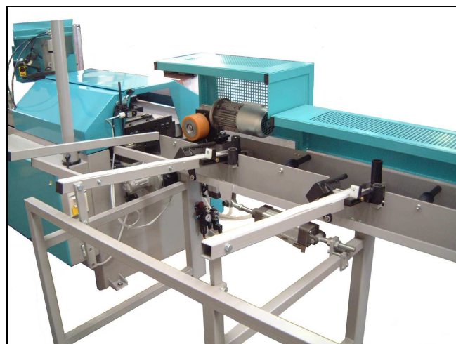
Baksida av maskin med fallmagasin och rulle för frammatning.
