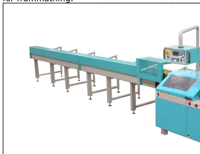
Vy framför maskin med magasin och skydd för oavsiktlig kontakt med frammatningsbanan.
